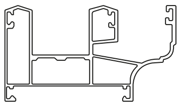
Code: E 104 پروفیل فریم ریلدار
