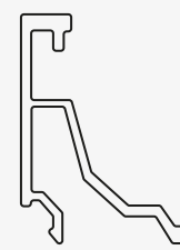
Code: E 109 پروفیل زوار دوجداره
