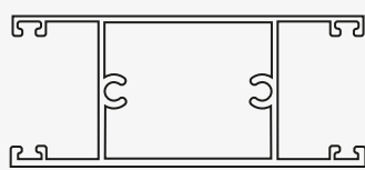
Code: E 102 پروفیل سپری کشویی
