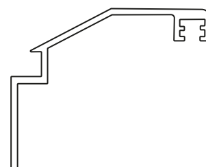
Code: E 112 روکوب ۳.۵
