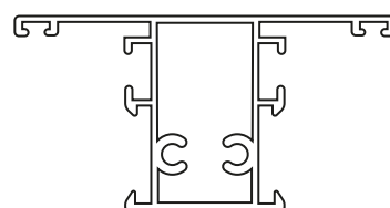
Code: E 119 سپری درب کوچک
